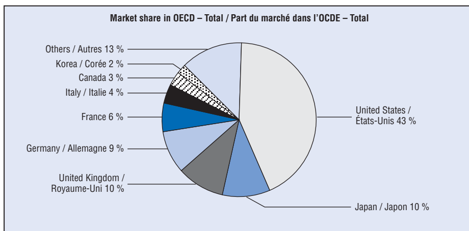
Figure I.1. Market share in OECD, 2004 / Part de marché dans l'OCDE, 2004 Direct gross premiums basis / Sur la base des primes brutes directes
